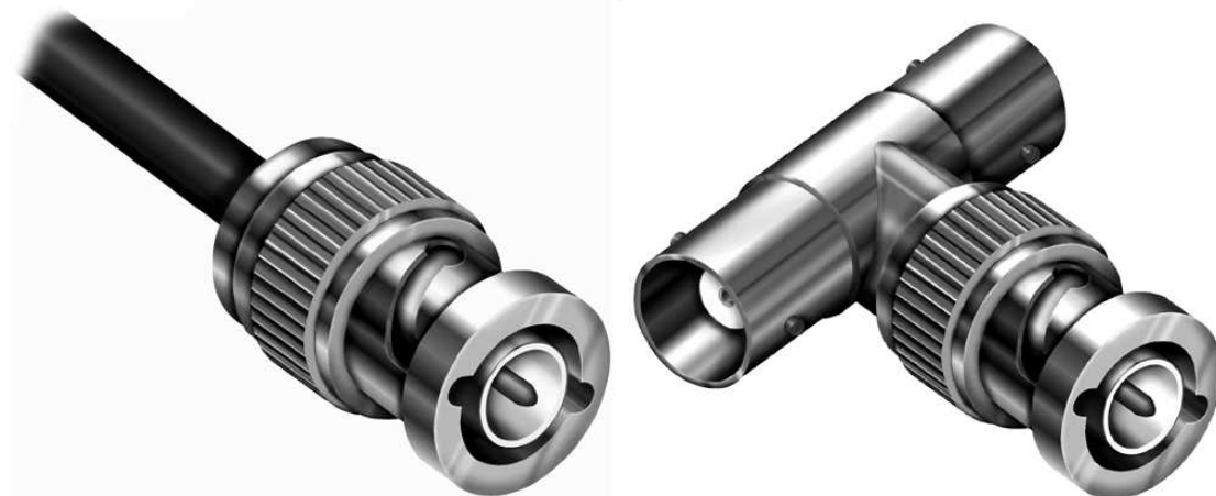
konektory BNC a BNC-T
